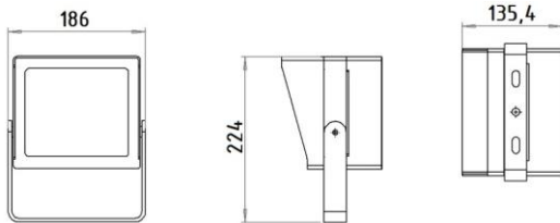
Рисунок 1 Светильник «L-point»
