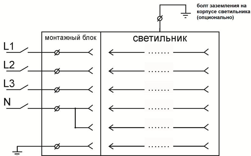
Рисунок 5 Схема подключения светильника
