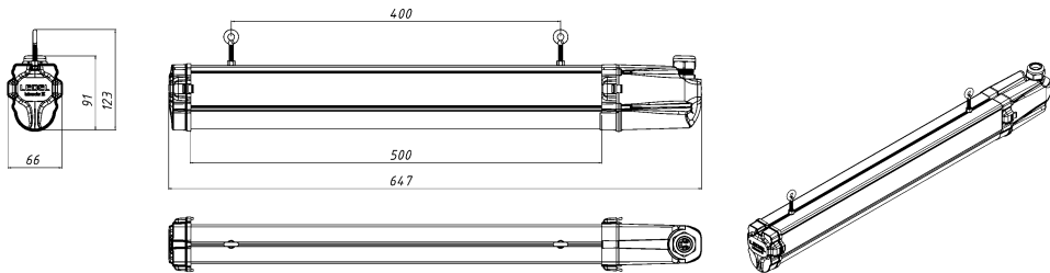
Рисунок 2 Светильник «L-trade II 20» с монтажным блоком
