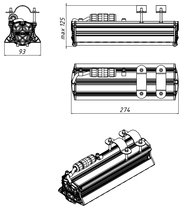
Рисунок 1 Габаритные размеры светильника «L-street 40 Turbine»
