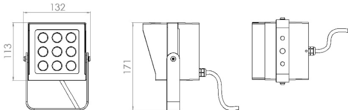
Рисунок 1 Светильник «L-point 9»
